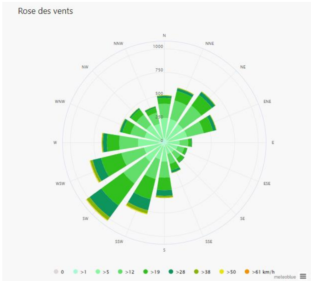
Normale de rose des vents station de Angers (meteoblue)
